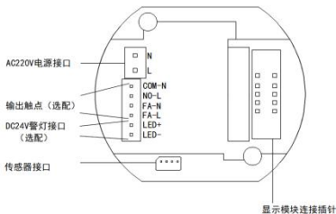
图 4-2 接线示意图
